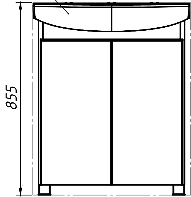
КЛЕРМОНТ Н70.00 СБ
